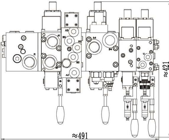
单泵双逻辑钻机阀
