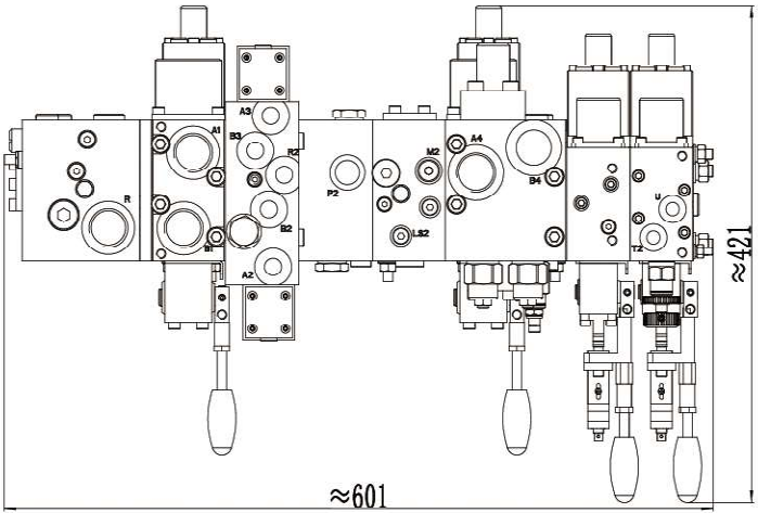
双泵双逻辑钻机阀
